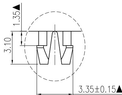
DETAILB SCALE: 2:1
