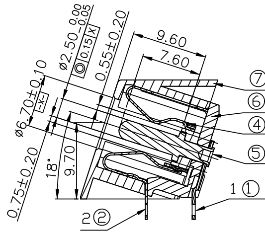
A-A 1:1
